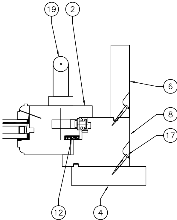
SECTION D-D
