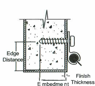
45° C-Channel
