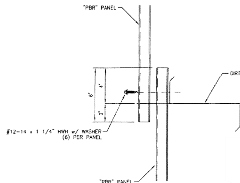
DETAIL #4 JAMB
