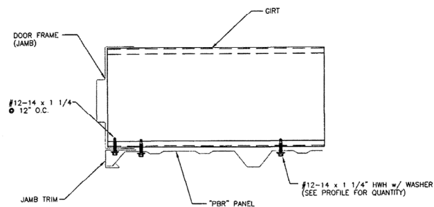
DETAIL #4 JAMB
