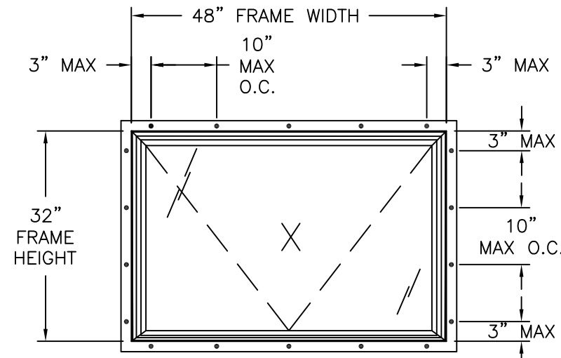
FIN INSTALLATION
