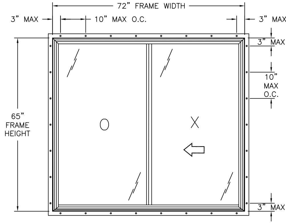
FIN INSTALLATION
