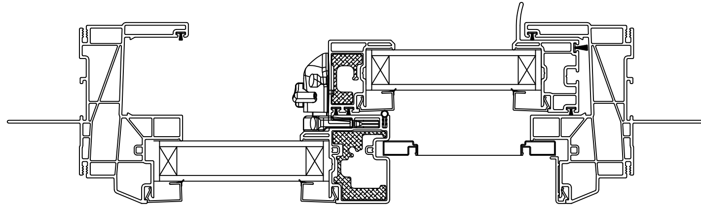
FIN HORIZONTAL CROSS SECTION
