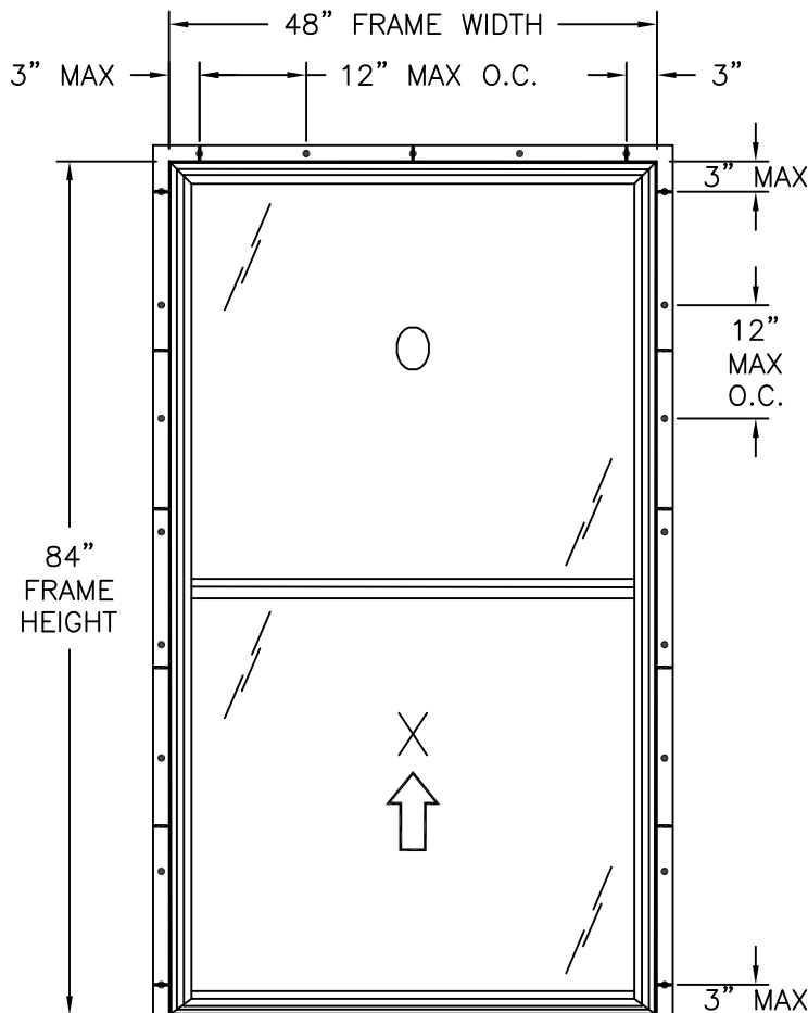
FIN INSTALLATION
