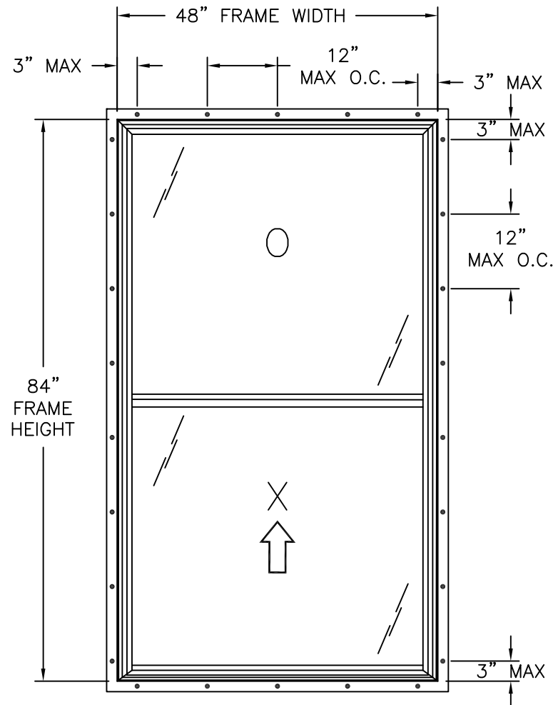
FIN INSTALLATION
