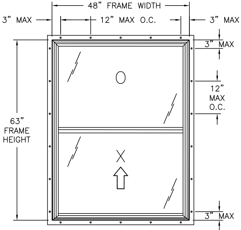
FIN INSTALLATION
