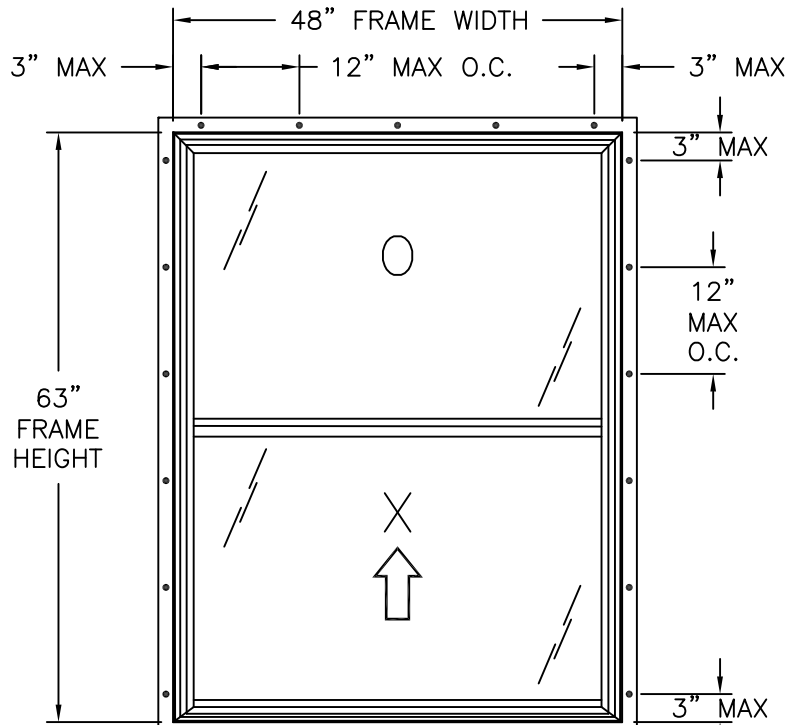
FIN INSTALLATION
