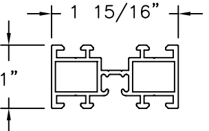
SLIDE BAR ALUMINUM 6063-T5
