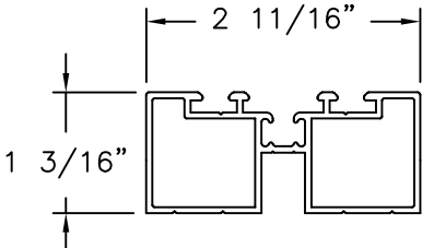
SIDE FRAME ALUMINUM 6063-T5
