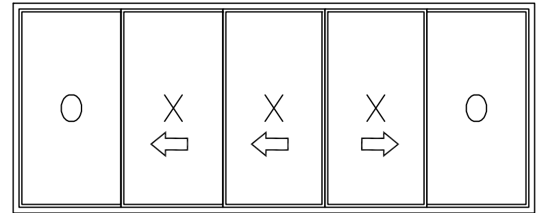
OXX/XO 3-TRACK
