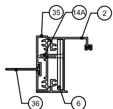
OPTIONAL FIN JAMB
