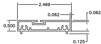
③⑤ NAIL FIN SUBFRAME
