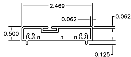
③⑤ NAIL FIN SUBFRAME
