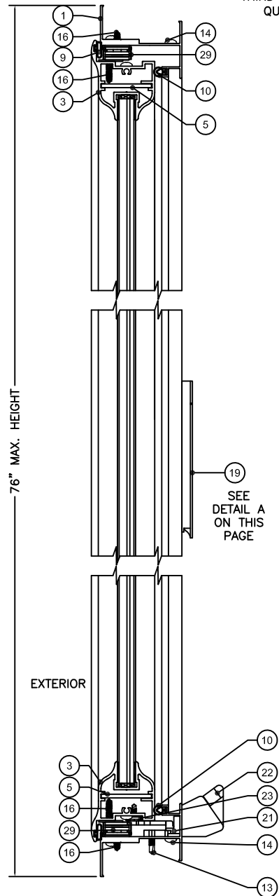
SECTION \frac{A}{3}
