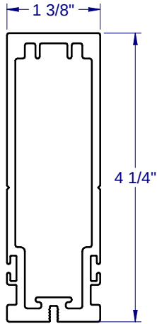
4" MULL BAR - 1759
