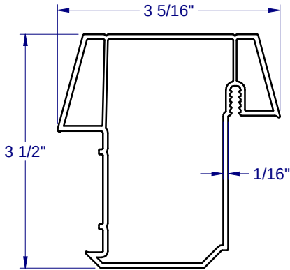
ASTRAGAL - 6272
