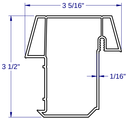
ASTRAGAL - 6272
