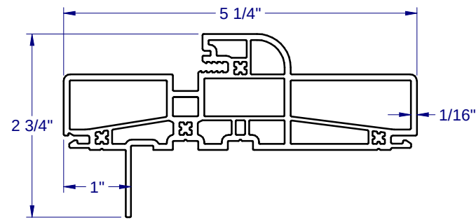
ALT. FIN FRAME - 6268
