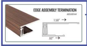
Edge Assembly Termination
