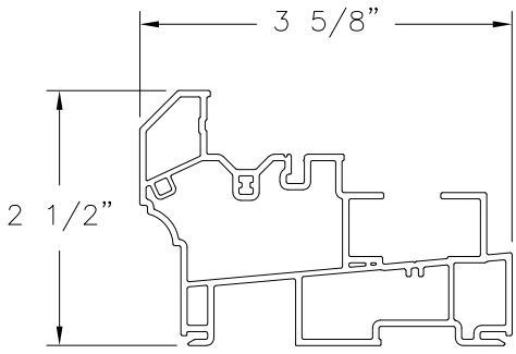
HEAD & JAMB FINLESS (10008686) RIGID PVC
