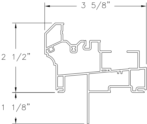
HEAD & JAMB FIN RIGID PVC
