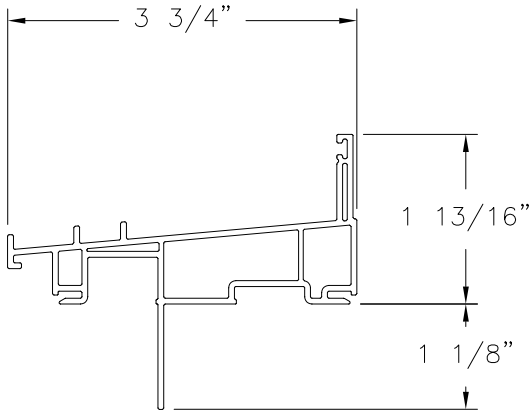
SILL FIN RIGID PVC
