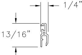
SILL RISER (10002916) RIGID PVC
