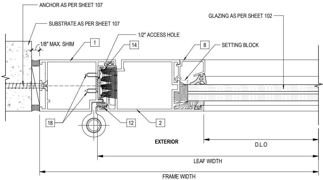
2 JAMB DETAIL-1 103 N.T.S
