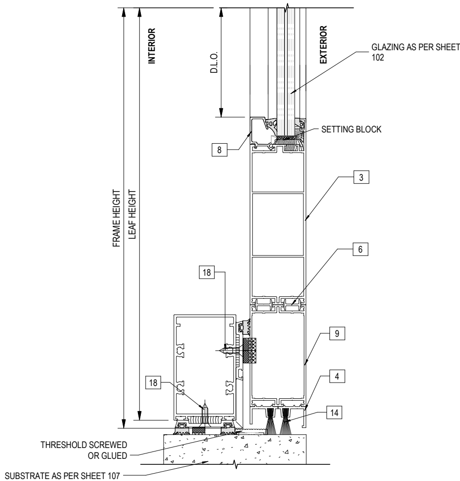
3 SILL DETAILS 103 N.T.S
