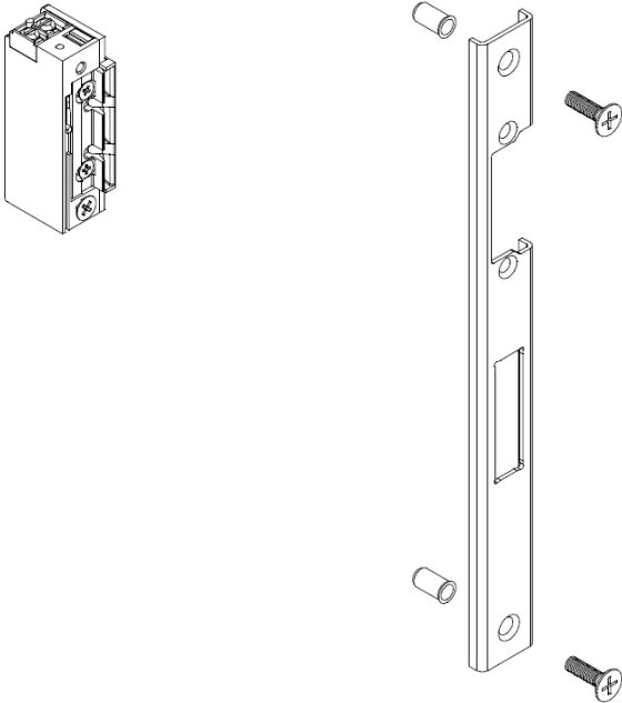
1 111 ELECTRIC STRIKE DETAILS N.T.S.
