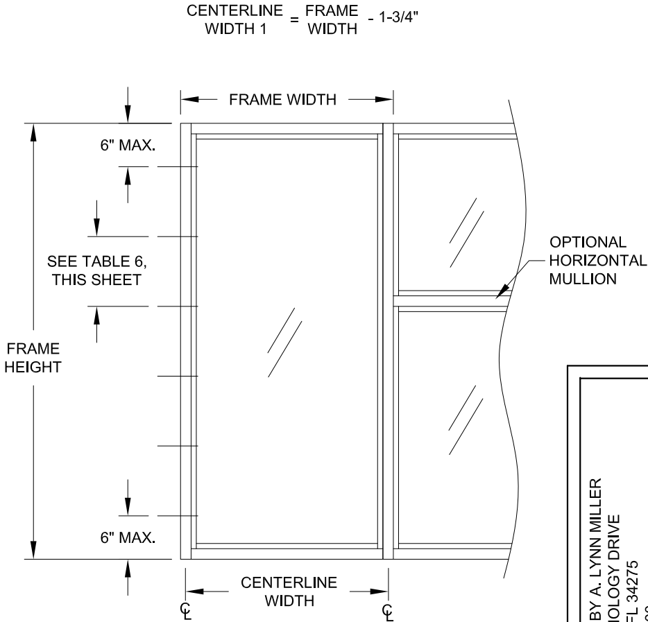
JAMB ANCHOR SPACING
