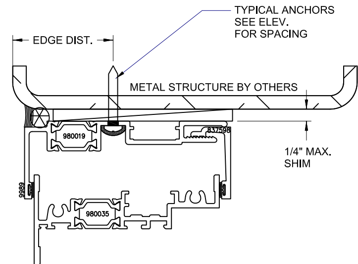
FRAME HEAD / JAMB
