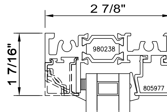
Optional Max. DLO Frame
