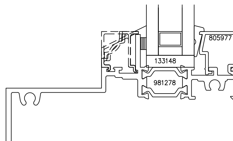
Optional SDH Frame
