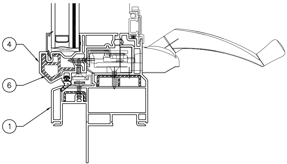
FIN FRAME
