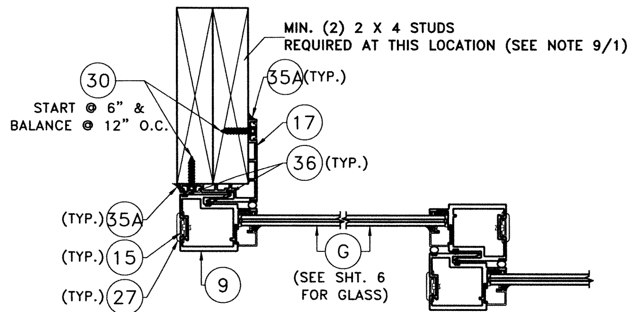
WOOD SUBSTRATE N.T.S.
