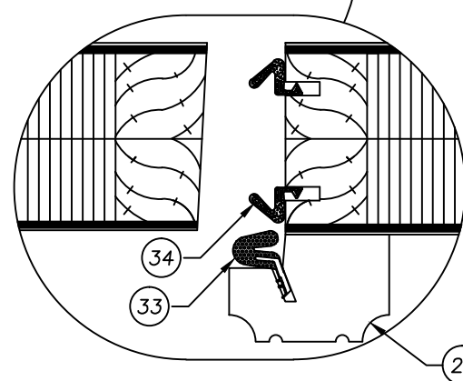
WEATHERSTRIP DETAIL DOOR D4-ACTIVE DOOR
