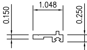
3 FRAME CAP
