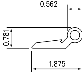
14 5 1/4" HINGE
