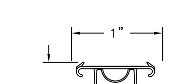
ENDURA ZAC SWEP WOOD G.46 MIN.
