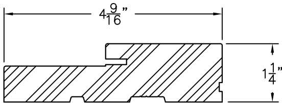
FRAME WOOD G.46 MIN.
