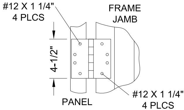
TYP. HINGE ANCHORAGE
