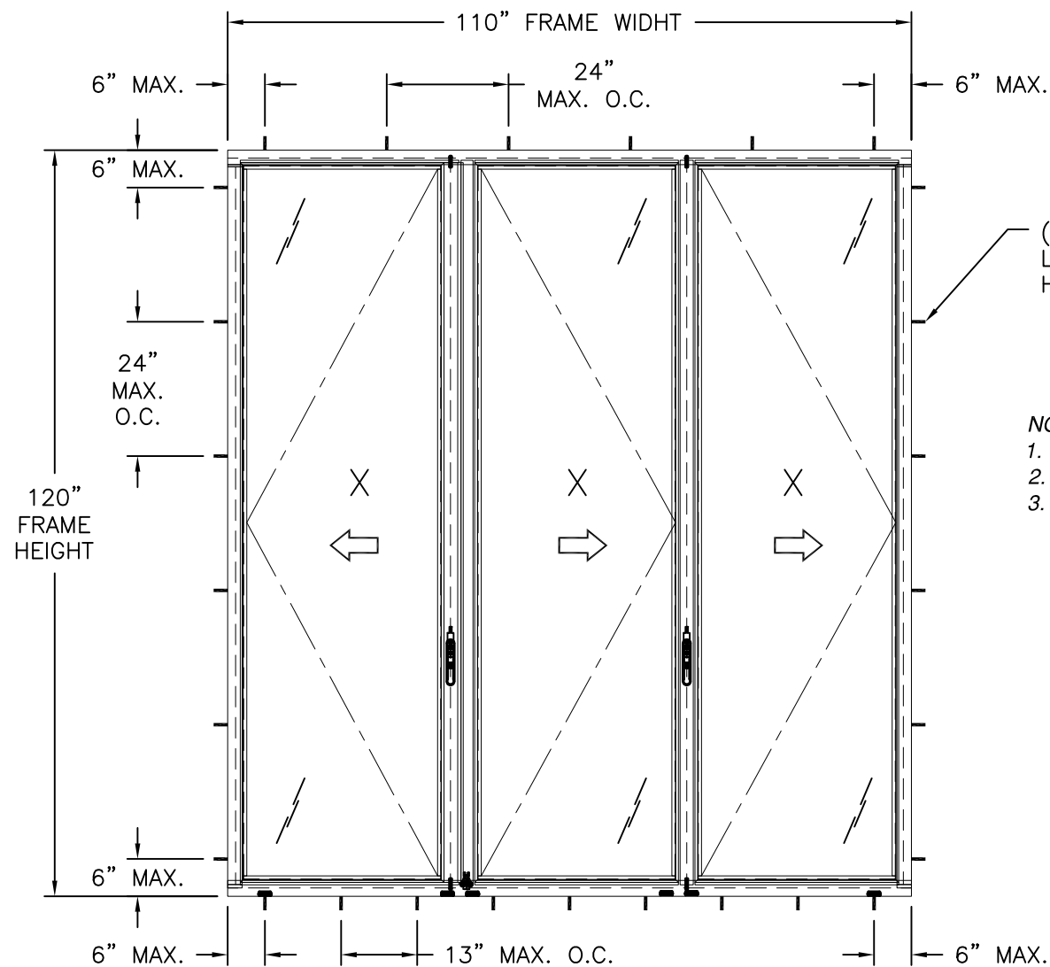
PALISADES S90 BI-FOLD DOOR INSWING 1L2R
