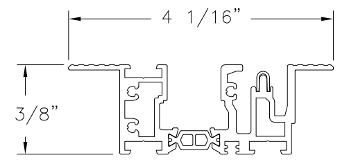
FLUSH SILL ALUMINUM 6063-T5
