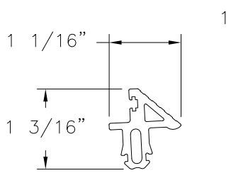
UNIVERSILL ALUMINUM 6063-T5
