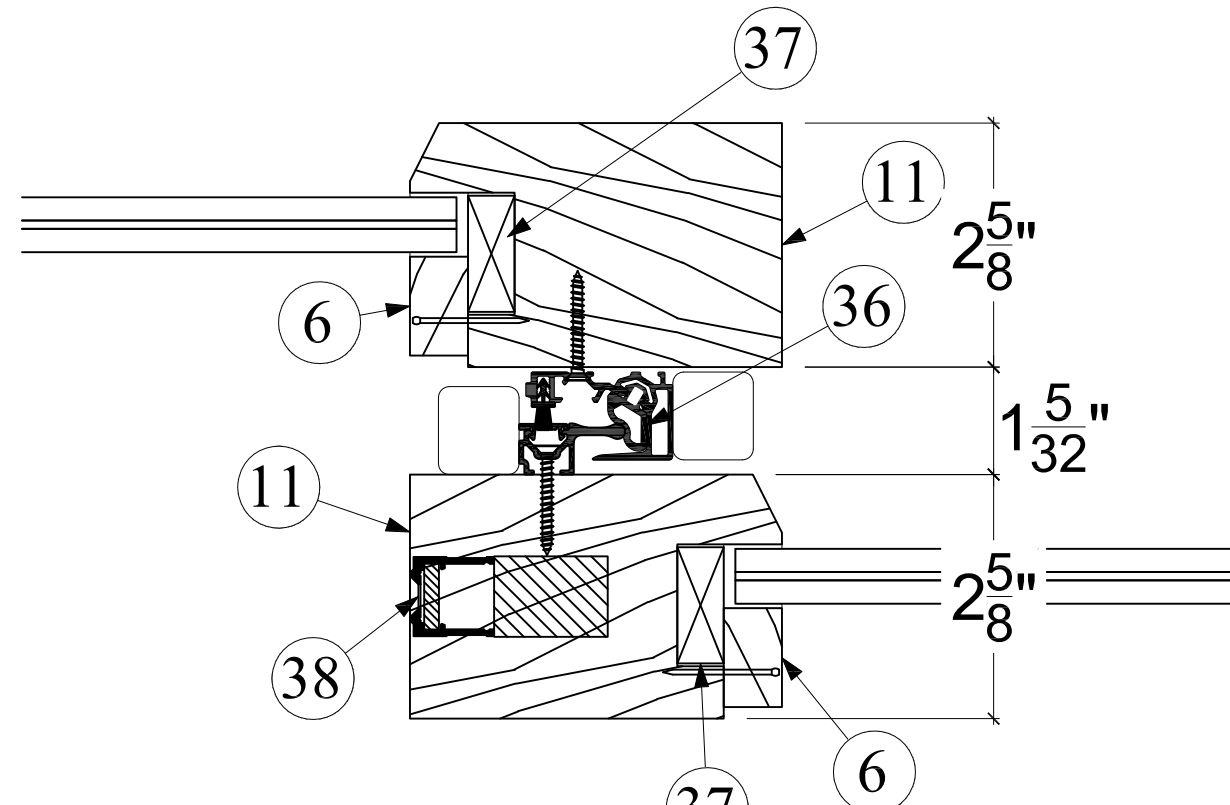
4B D5 FFI INTERLOCK
