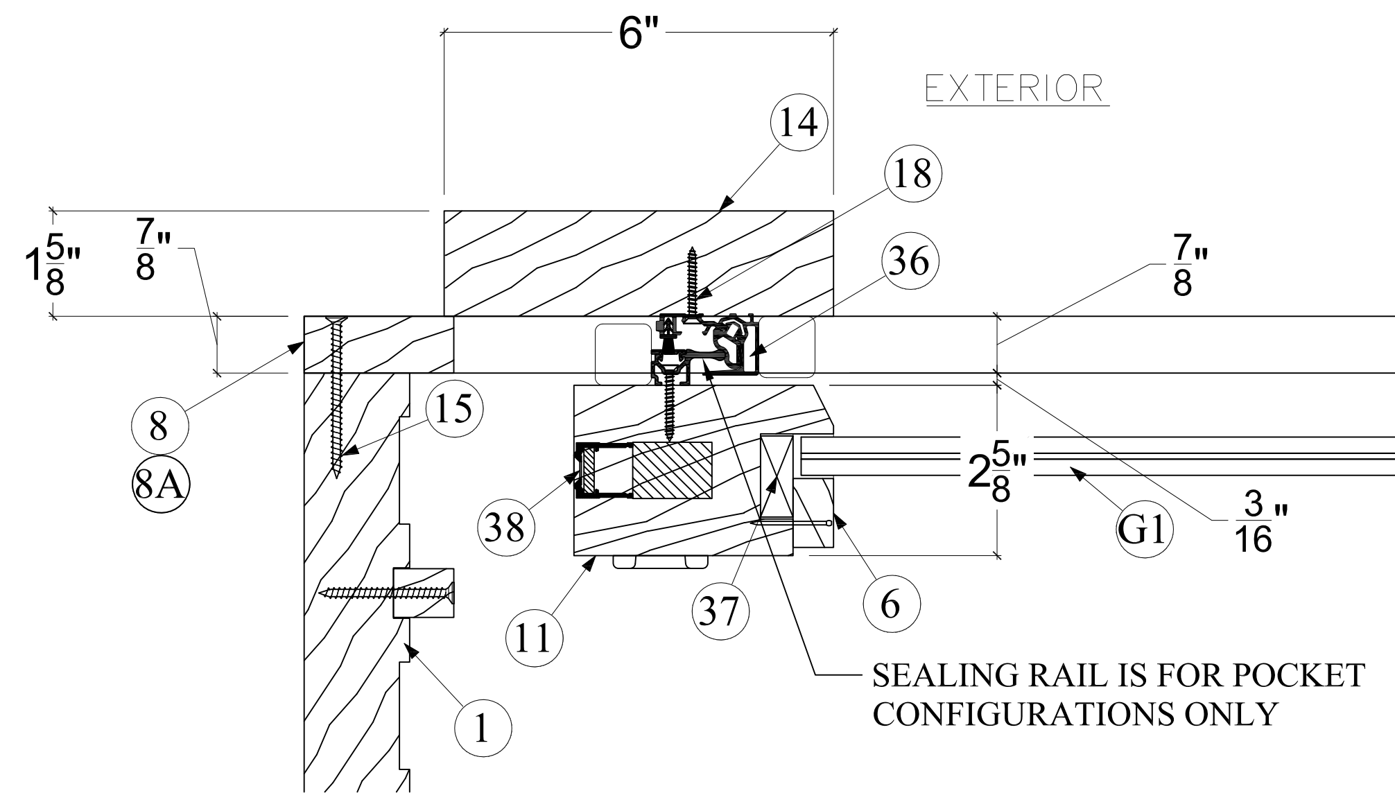
2 D5 POCKET JAMB
