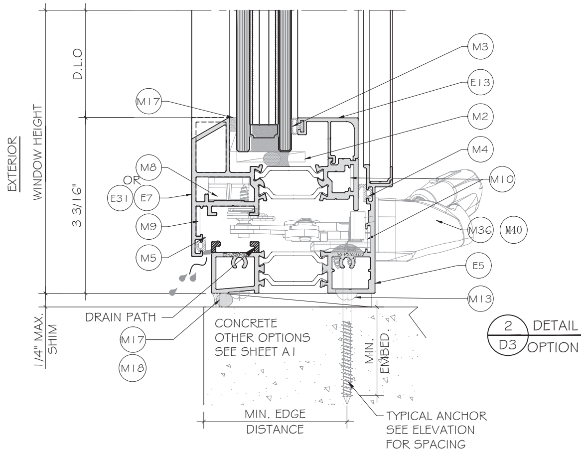
2 D3 DETAIL
