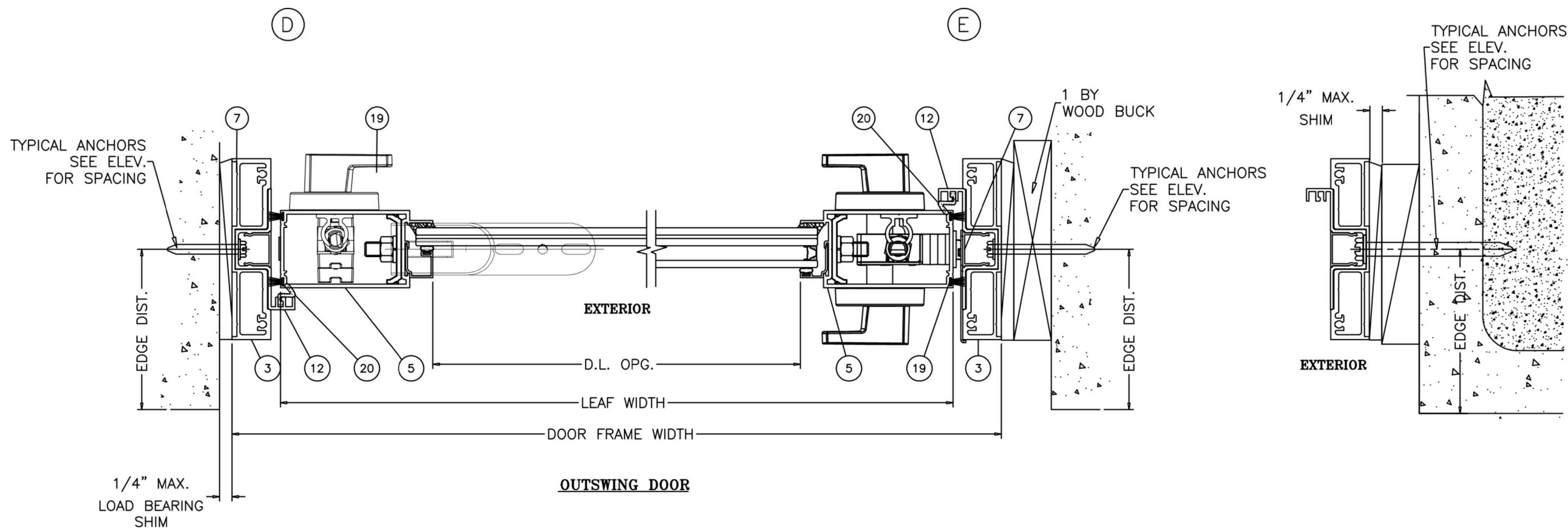
DOOR DETAILS
