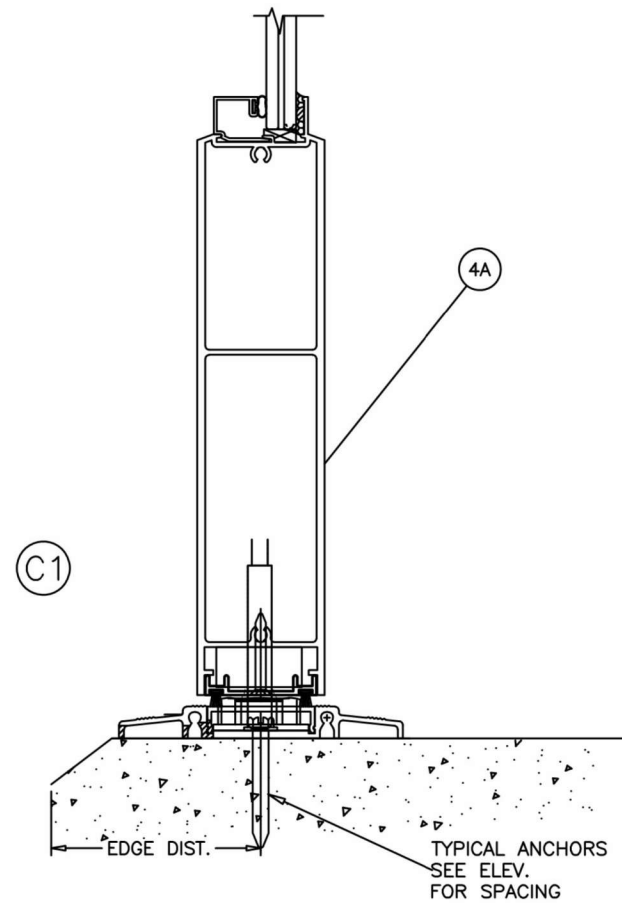
DOOR DETAILS
