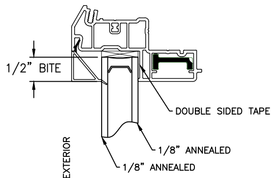
IG GLAZING GL1
