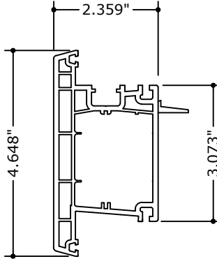
② DOOR T-SASH 541150
