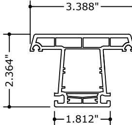
③ T-MULLION 554091
