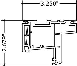
1 FIXED FRAME 601205
