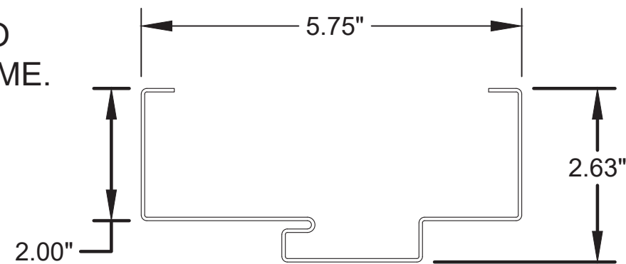
2 ) HOLLOW METAL FRAME JAMB
