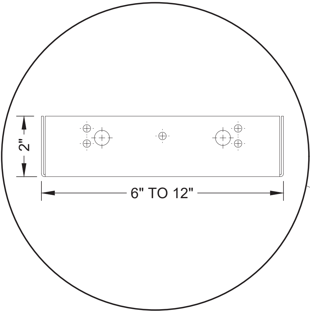
SUBFRAME (ITEM 4) END FABRICATION
