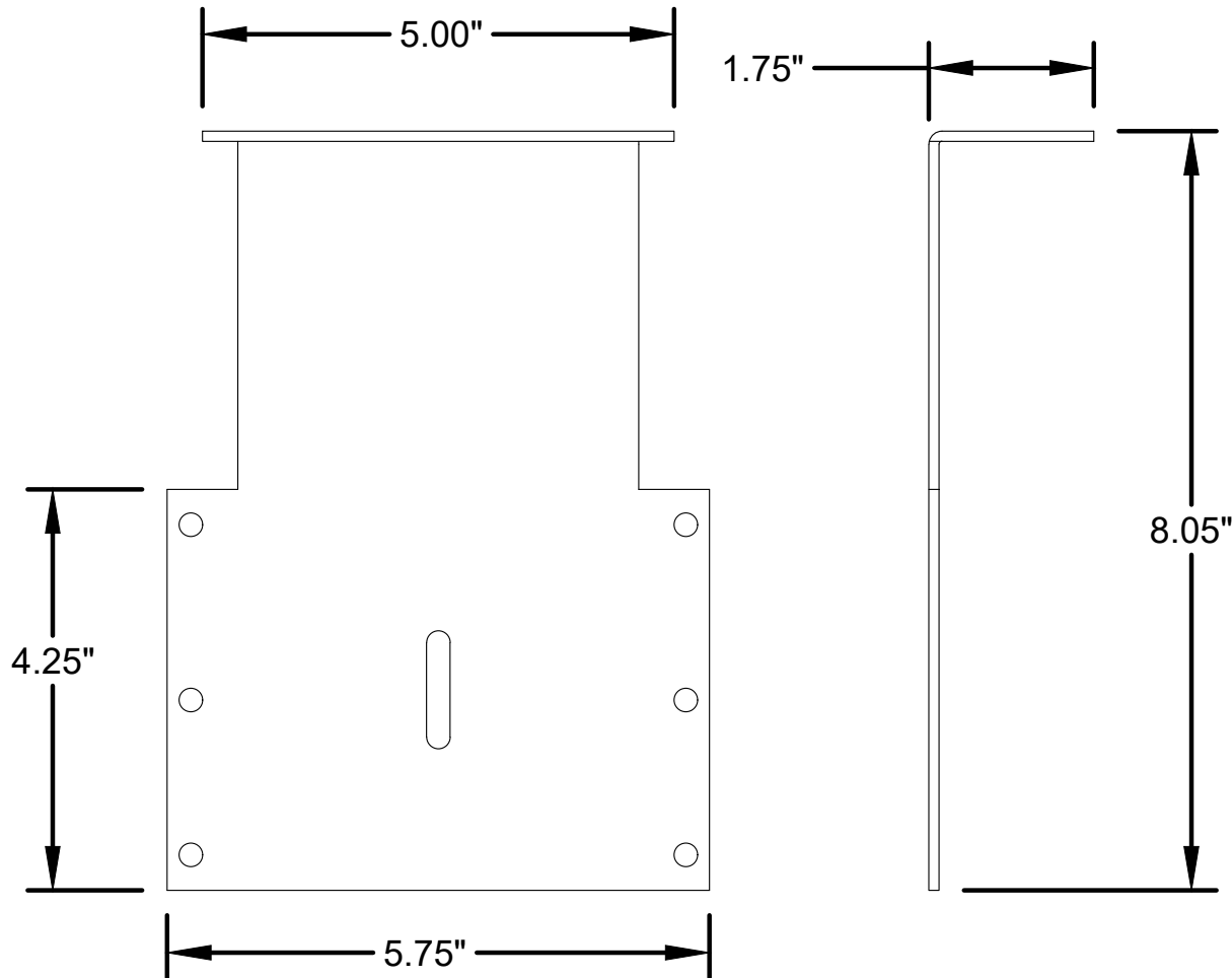
2 HOLLOW METAL FRAME JAMB
