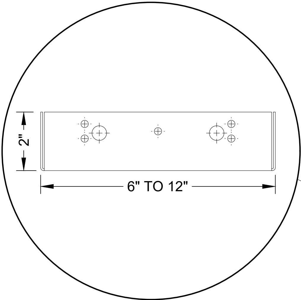
SUBFRAME (ITEM 4) END FABRICATION
