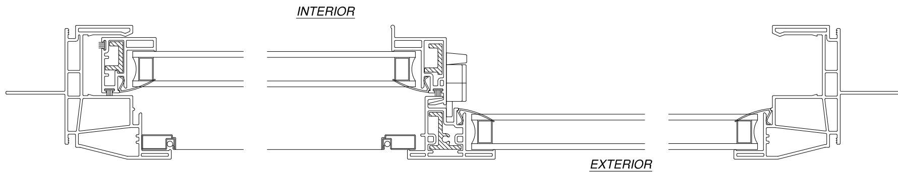
HORIZONTAL CROSS SECTION FIN FRAME
