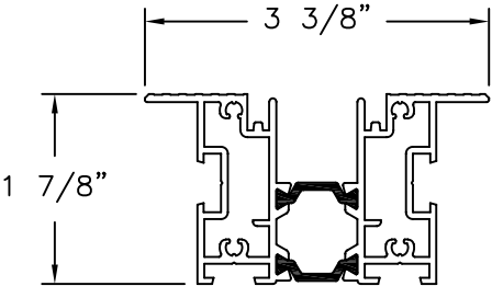
FLUSH SILL ALUMINUM 6063-T5
