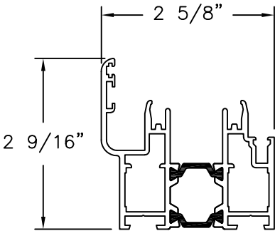
HEAD & JAMB FRAME ALUMINUM 6063-T5
