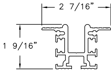
FLUSH SILL ALUMINUM 6063-T5
