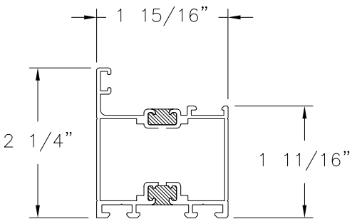
DOOR FRAME ALUMINUM 6063-T5
