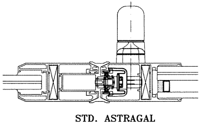
STD. ASTRAGAL
