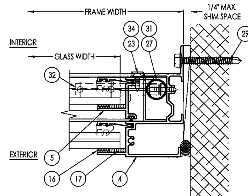
D FRAME JAMB 2
