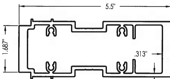
10 MULLION (SUN-18)
