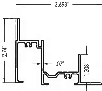
4 FRAME JAMB (SUN-254)
