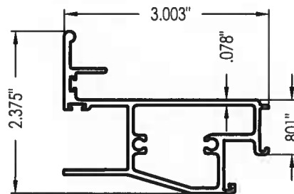
5 SASH JAMB (SUN-255)
