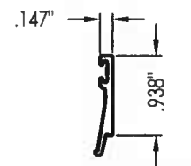
8 GLAZING BEAD (SUN-258)
