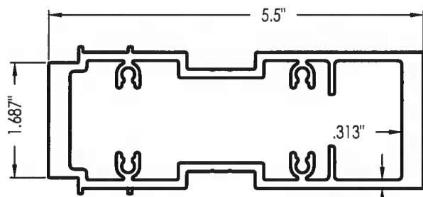
10 MULLION (SUN-18)
