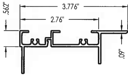
1 HEAD (SUN-251)
