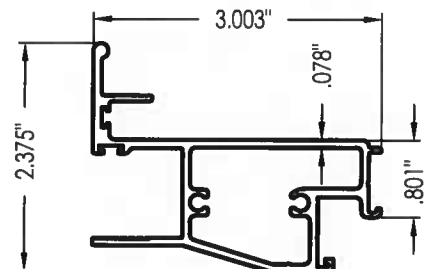
5 SASH JAMB (SUN-255)
