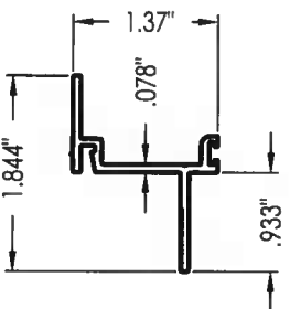
5 SASH JAMB (SUN-255)
