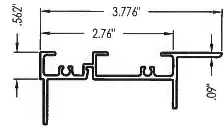
1 HEAD (SUN-251)
