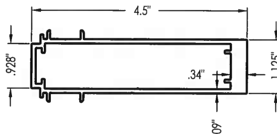
10 MULLION (SUN-264)
