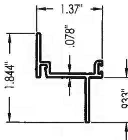
5 SASH JAMB (SUN-255)
