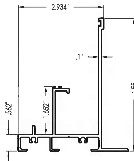
3 FRAME SILL (SUN-253)
