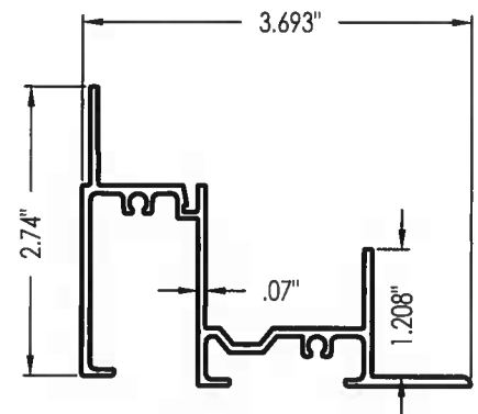
4 FRAME JAMB (SUN-254)
