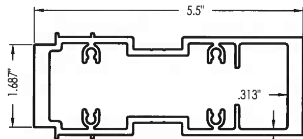
10 MULLION (SUN-18)
