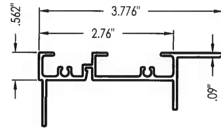
1 HEAD (SUN-251)
