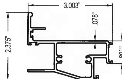
5 SASH JAMB (SUN-255)
