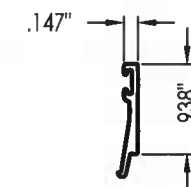
8 GLAZING BEAD (SUN-258)
