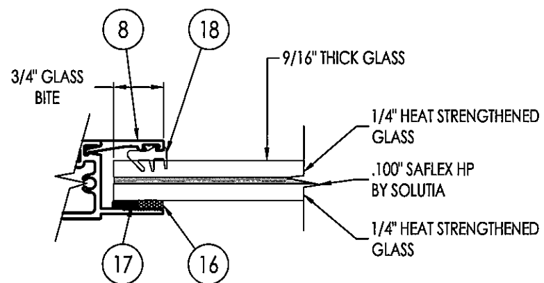
G2 GLAZING DETAIL
