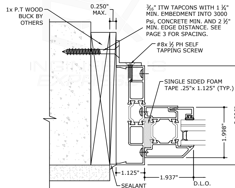
6.3 JAMB DETAIL
