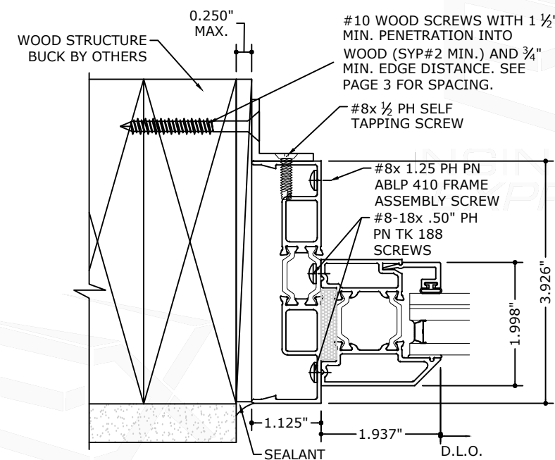
6.4 JAMB DETAIL
