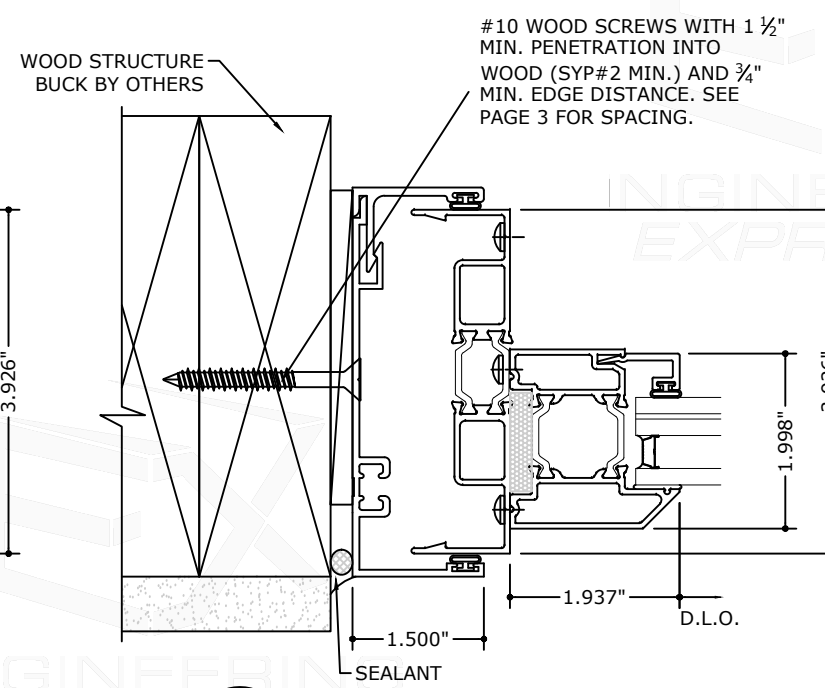
7.4 JAMB DETAIL
