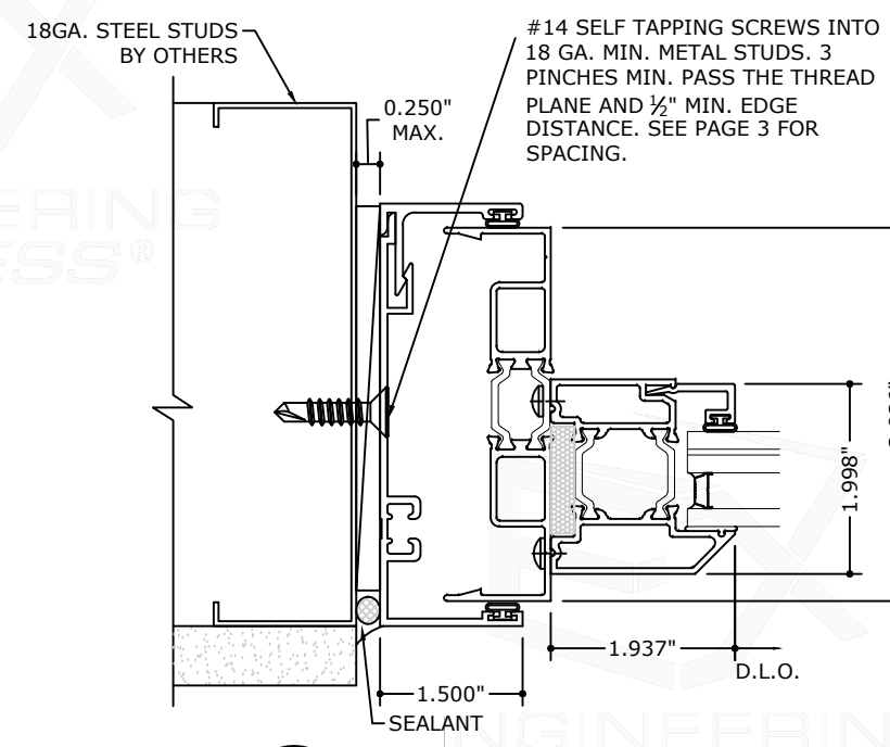
7.5 JAMB DETAIL
