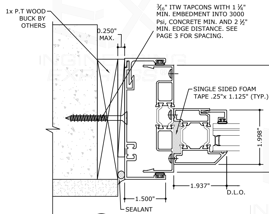
7.3 JAMB DETAIL
