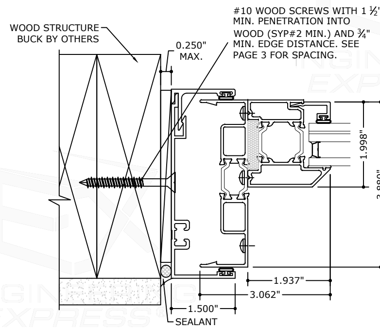
7.1 JAMB DETAIL
