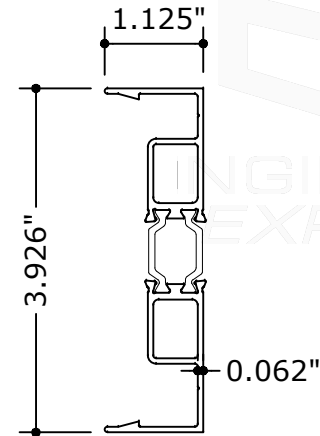
3 FRAME JAMB
