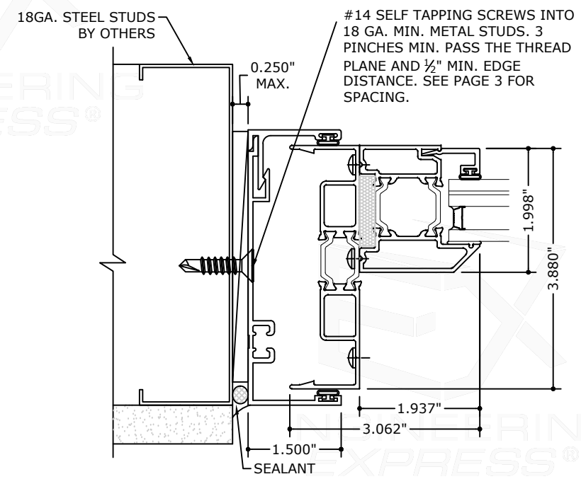
7.2 JAMB DETAIL
