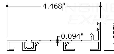
4 JAMB SASH
