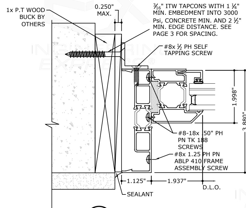
6 JAMB DETAIL
