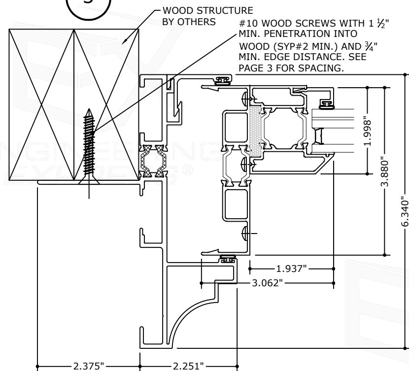
3.1 JAMB DETAIL
