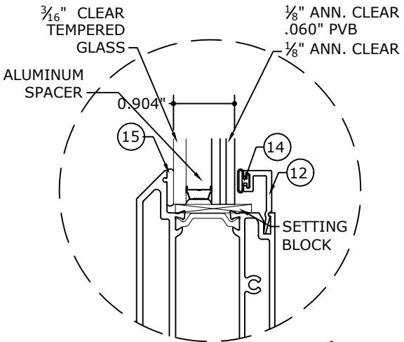
GLASS TYPE G2 GLAZING DETAIL N.T.S.
