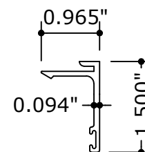
3 FRAME JAMB
