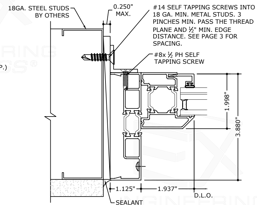
6.2 JAMB DETAIL
