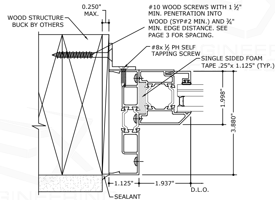
6.1 JAMB DETAIL
