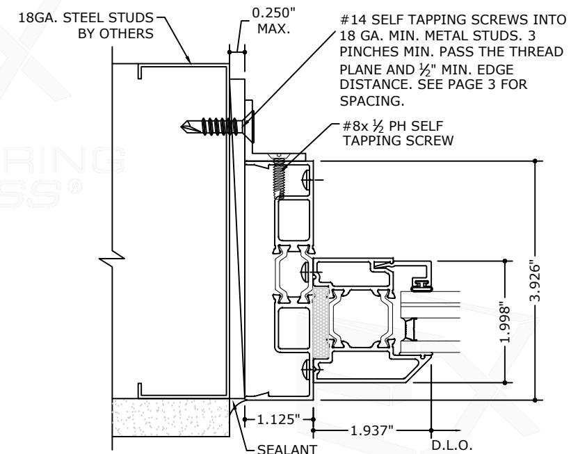
6.5 JAMB DETAIL
