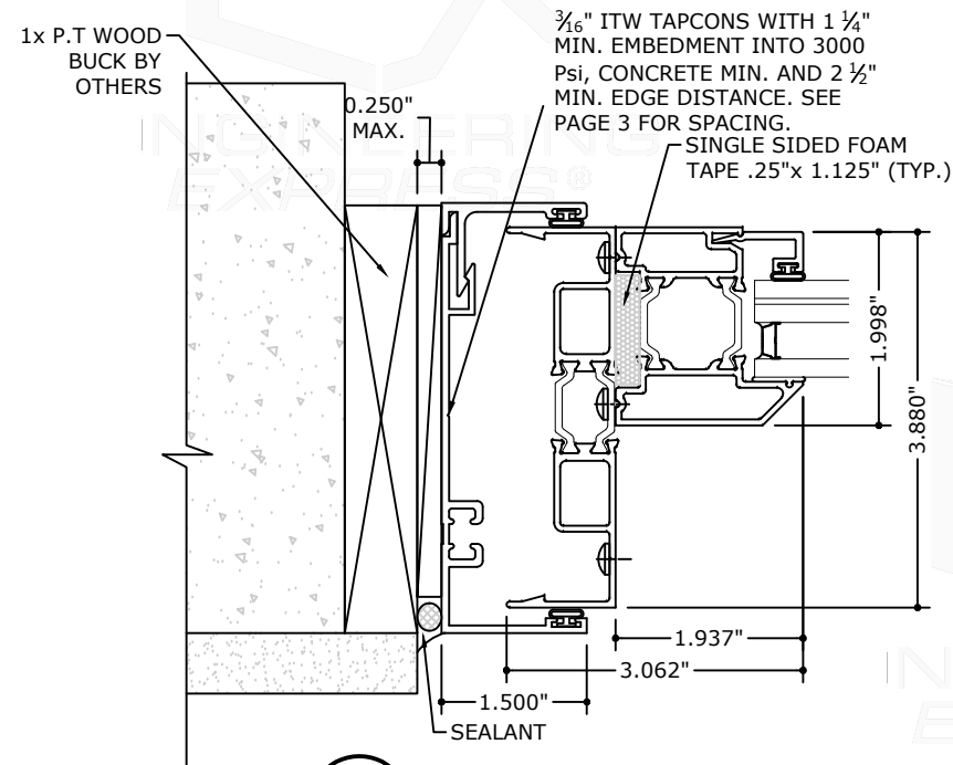
7 JAMB DETAIL
